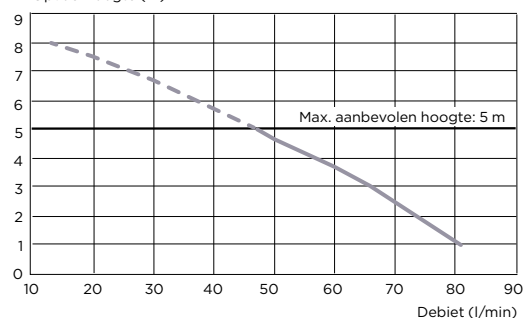
Opvoerhoogte (m)
