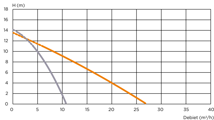
SANIPUMP® vortex
