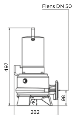
Draagbare montage wijze
