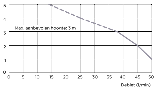
Opvoerhoogte (m)
