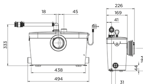
SANIACCESS® 3
