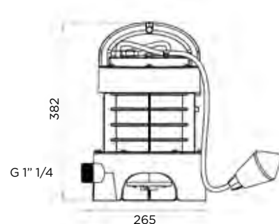
SANIPUMP® vermaler
