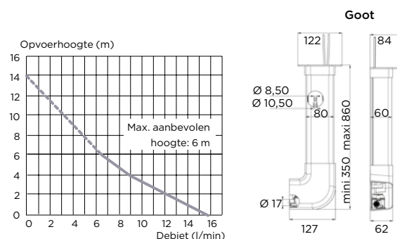
Sanicondens Clim mini (geleverd inclusief bevestigingssteun)
